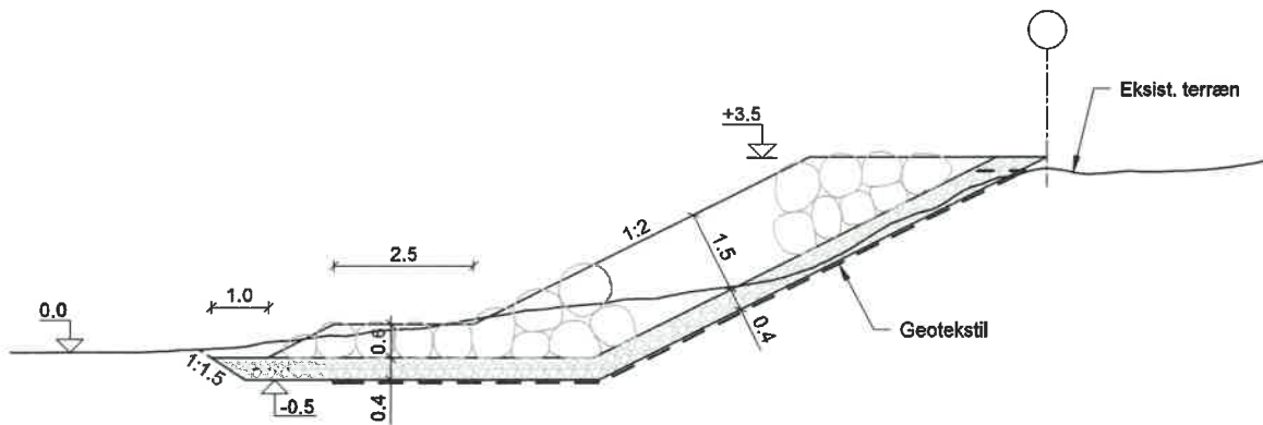
PRINCIPSNIT , 1:100 Delstrækning A
