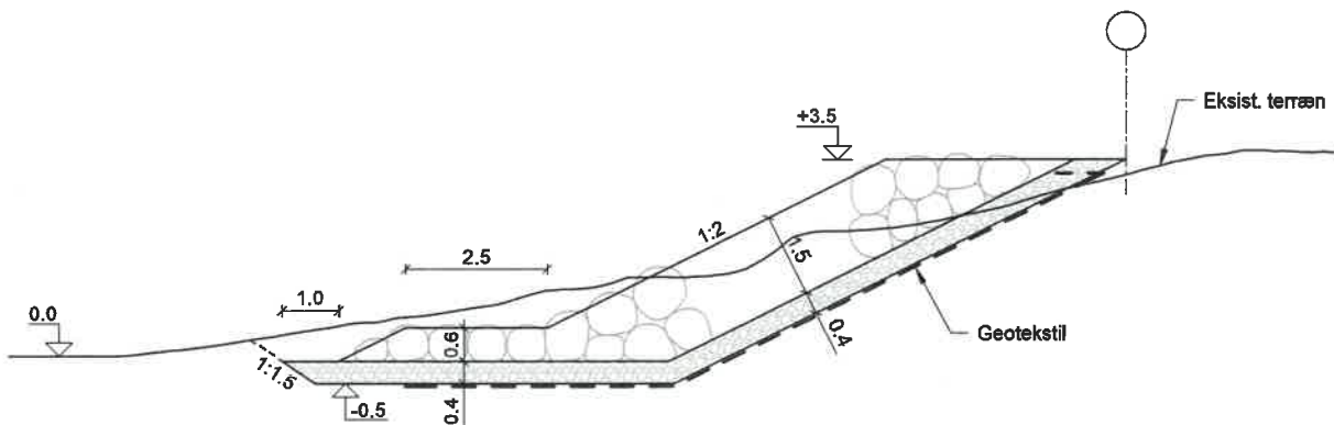
PRINCIPSNIT , 1:100 Delstrækning B
