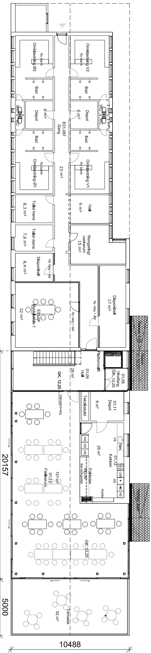
Stueplan
